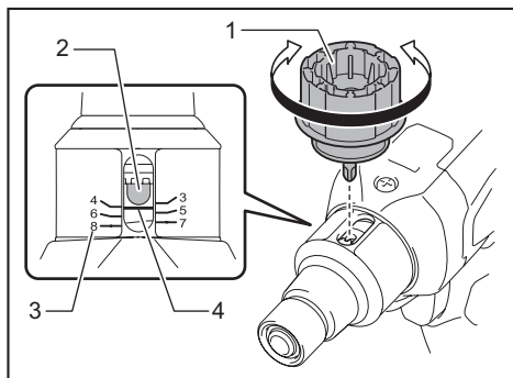
► 1. Chave de ajuste 2. Furo para a chave de ajuste 3. Escala 4. Linha amarela
