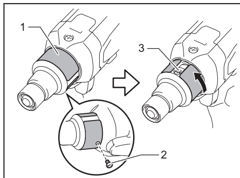
► 1. Anel 2. Parafuso 3. Furo
